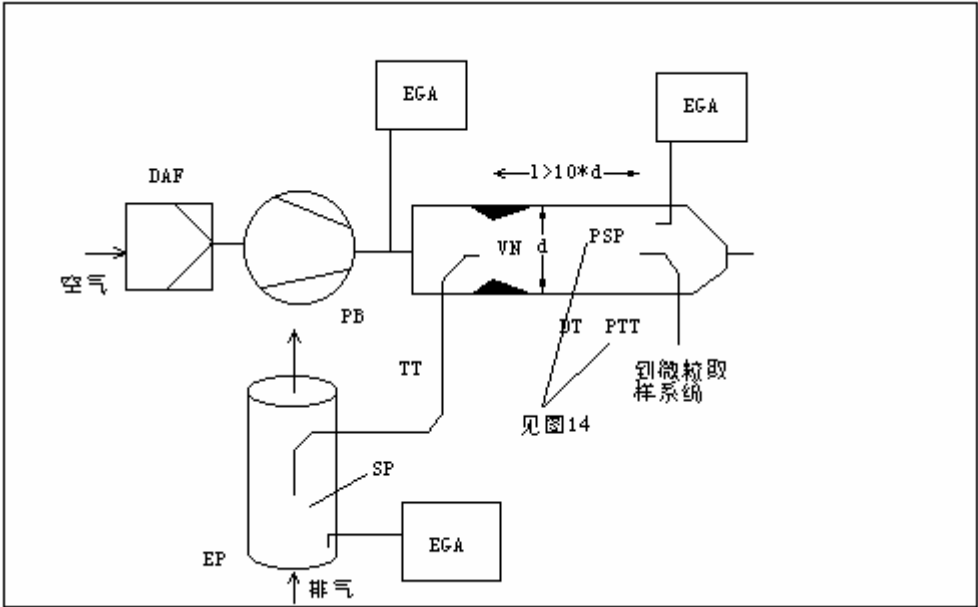
图 8 带单文丘里管，浓度测量，部分流取样的部分流稀释系统
