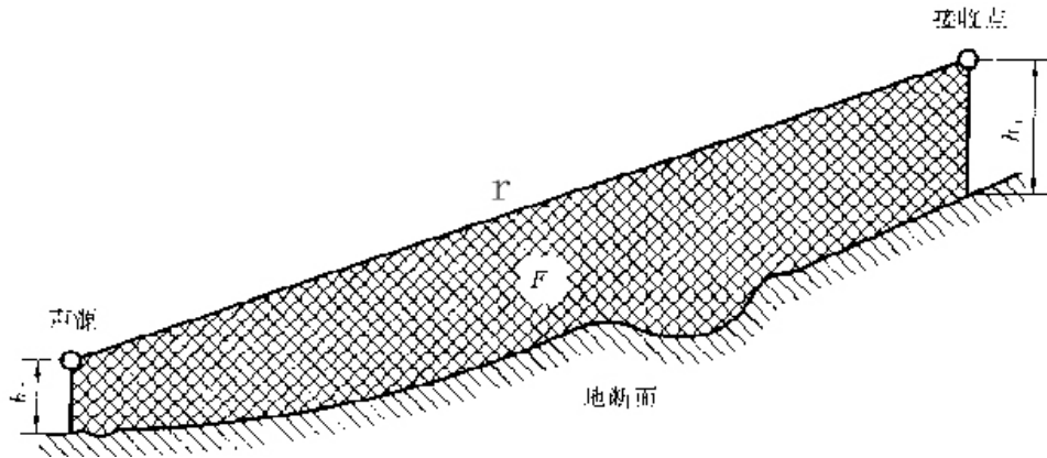
图 5 估计平均高度 h_m 的方法
