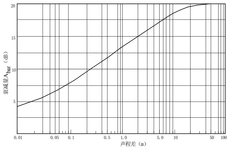
图 A.5 噪声衰减量 A_{\bar{a}} 与声程差 \delta 关系曲线 (f=500Hz)
